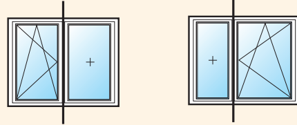
Fenster 2-flügelig Fest/DK symmetrisch oder asymmetrisch
